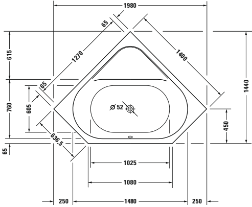
# 700137 00 0 00 0000, 1400 x 1400 mm Einbauversion
