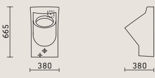
Elektronik-Urinal Architec für Netzanschluss # 0820360093 Seite: Abb. 87, TZ 162
