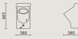
Elektronik-Urinal Architec für Batterieanschluss # 0820360000 Seite: Abb. 87, TZ 162
