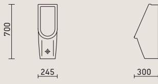
Urinal Starck 3 # 082725 Seite: Abb. 88, 91, TZ 162
