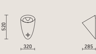
Urinal Starck 1 # 083432 Seite: Abb. 91, TZ 163
