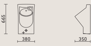
Elektronik-Urinal Architec für Netzanschluss # 0818360093 Seite: Abb. 86, TZ 162
