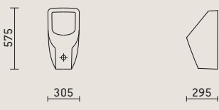
Urinal D-Code # 082830 Seite: Abb. 90, TZ 162
