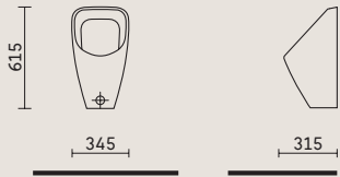
Urinal Duraplus # 083036 Seite: Abb. 91, TZ 163
