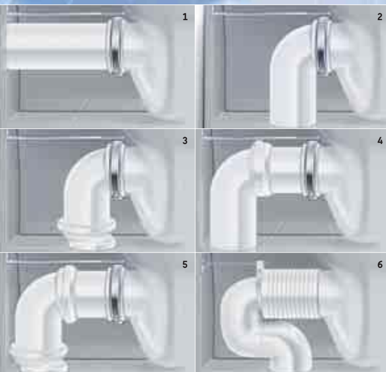
Abb. 1 Abgang waagrecht
