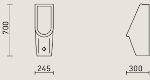
Urinal Starck 3 # 082625 Seite: TZ 162
