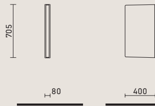
Urinal-Trennwand # 850000 Seite: Abb. 89, TZ 164
